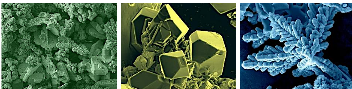
Slike elektronske vrstične mikroskopije ekstrahiranih faz iz aluminijevih zlitin
